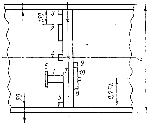
Схема вырезки образцов для испытаний ( b — ширина листа)
